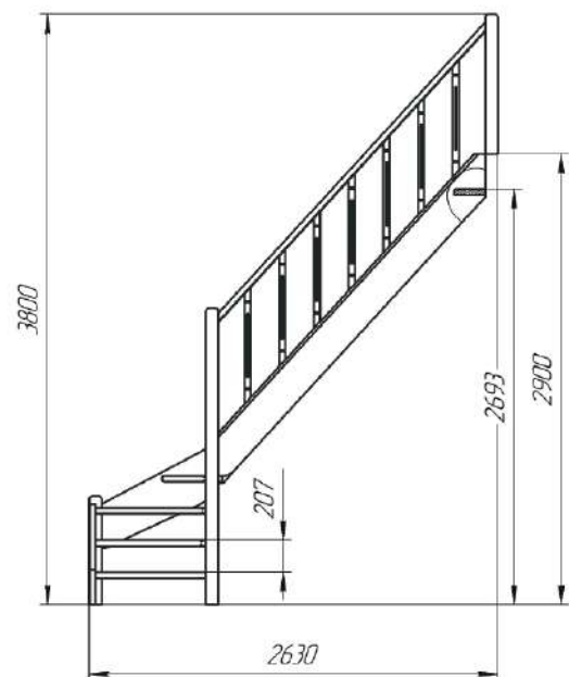
Рисунок 1. Лестница внутриквартирная ЛЕС-07.
